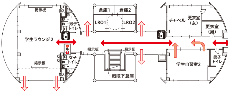
1 階平面図
