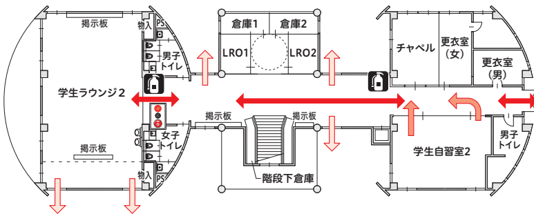
1 階平面図
