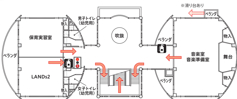
2 階平面図
