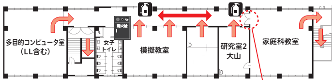
3階平面図
